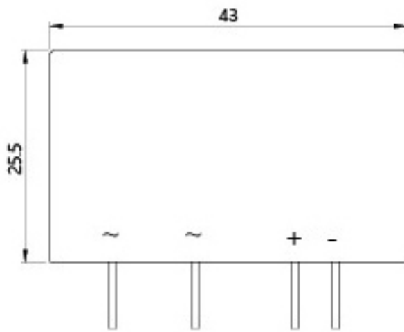
尺寸图
