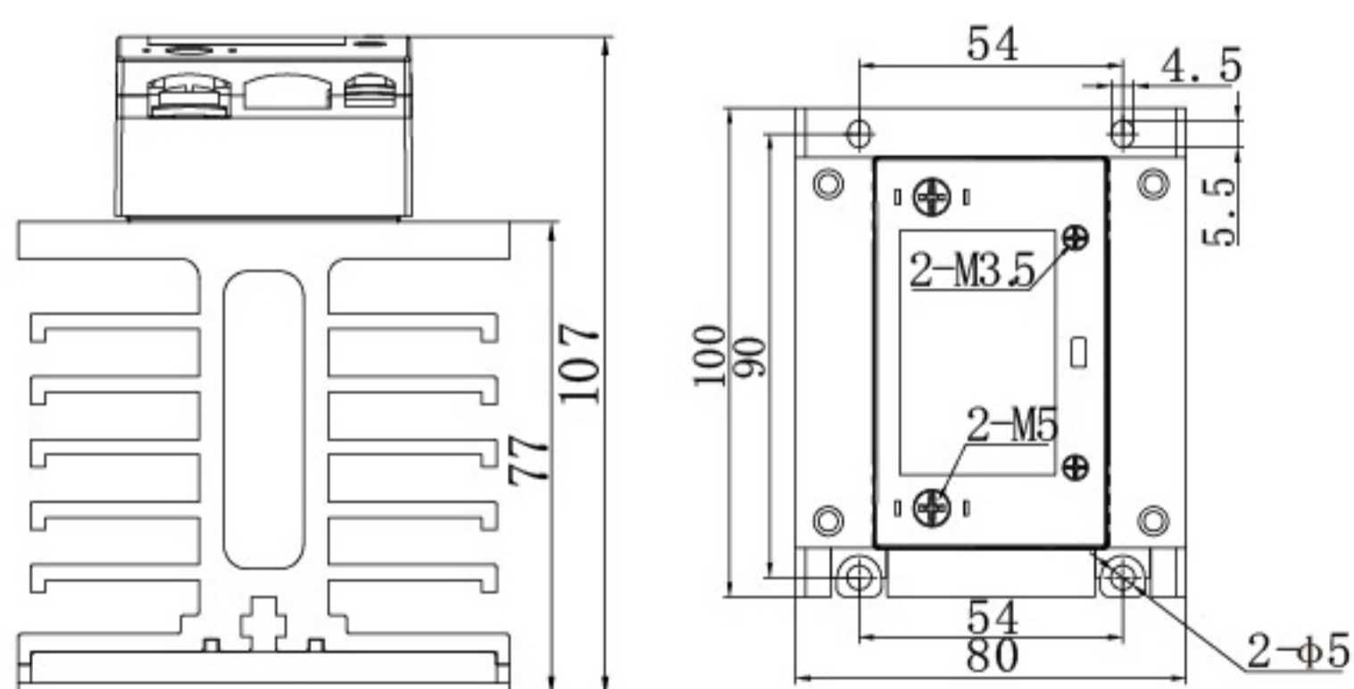
尺寸图
