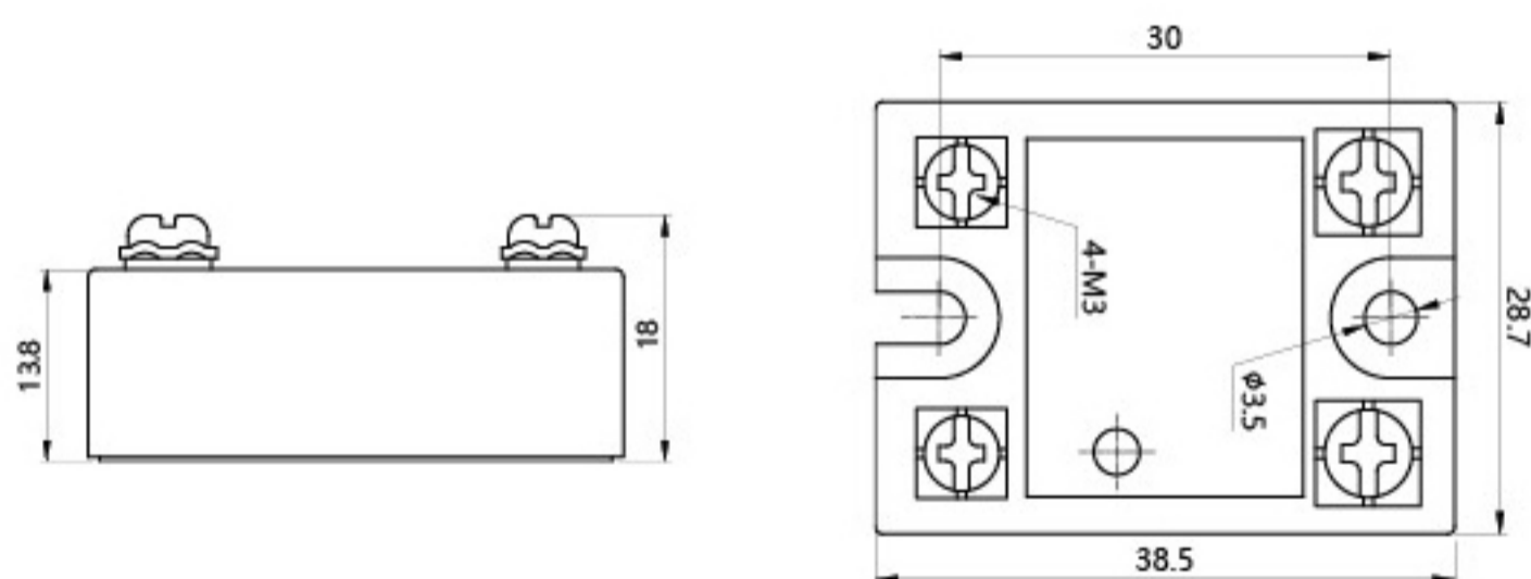
尺寸图
