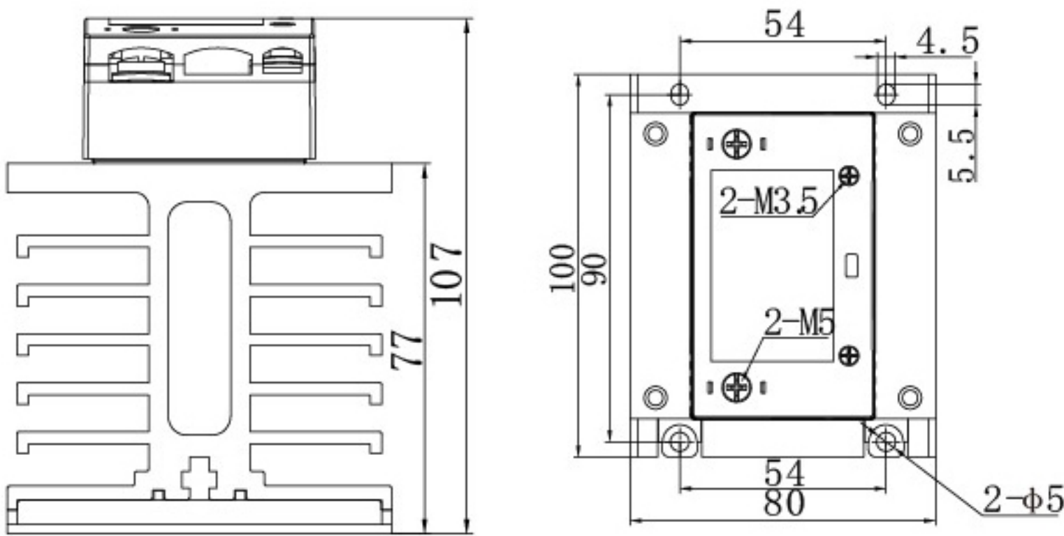
尺寸图
