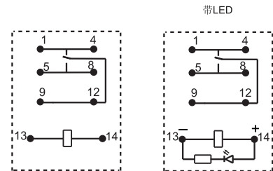
接线图(底视图)
